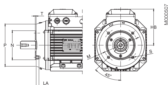
Flange-mounted motor, small flange; IM B14 (IM 3601)
